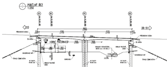
Řez mostem u IKEA do Robotnice
