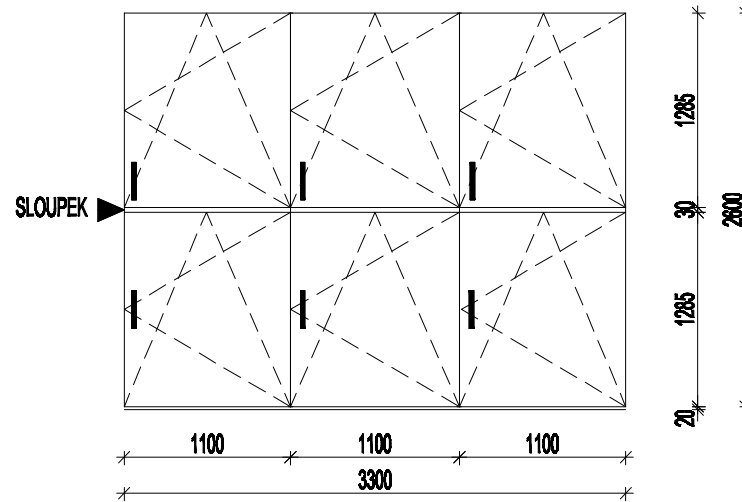
OKNO - TYPU 2, 8KS
