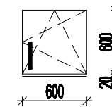
OKNO - TYPU 5, 3KS
