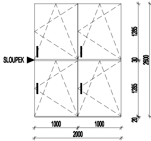
OKNO - TYPU 1, 14KS
