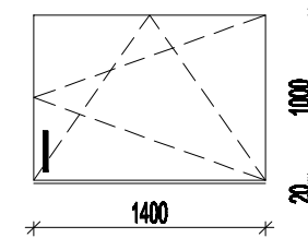
OKNO - TYPU 3, 12KS
