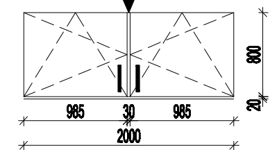
OKNO - TYPU 6, 2KS
