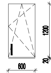
OKNO - TYPU 4, 1KS
