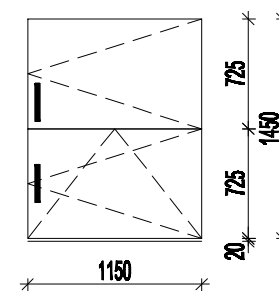
OKNO - TYPU D, 4KS
