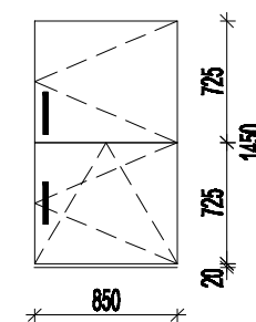
OKNO - TYPU E, 2KS
