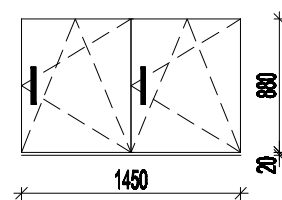
OKNO - TYPU C, 4KS
