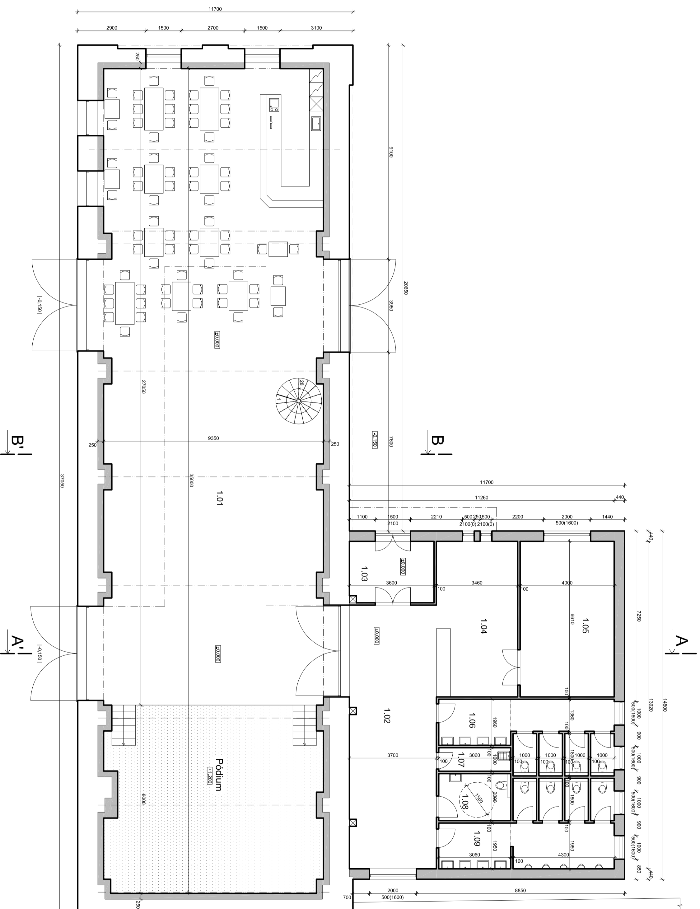
LEGENDA MÍSTNOSTÍ 1.NP
